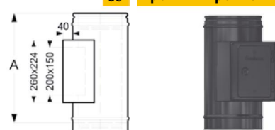
6с Тройник прочистки для твердого топлива
