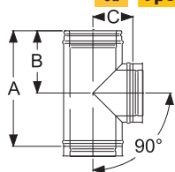
6a Тройник 90°
