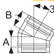
7c Отвод 30°
