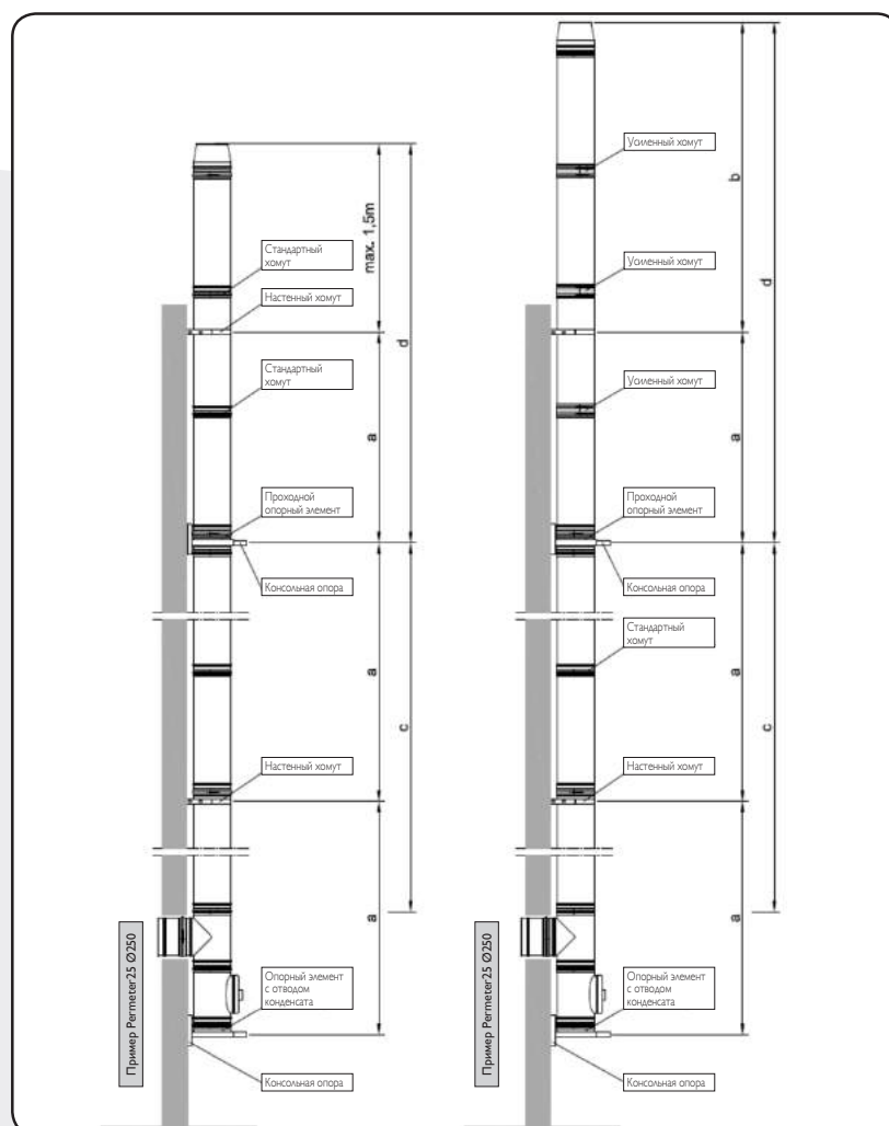
PERMETER25 Ø130-Ø250
