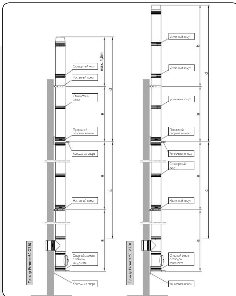
PERMETER50 Ø130-Ø250
